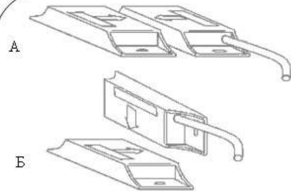
Рисунок 2. Варианты крепления датчиков
