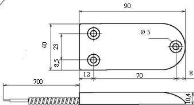
Рисунок 4. Габаритные и присоединительные размеры Напольного исполнения извещателя
