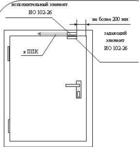
Рисунок 5. Пример установки извещателя для охраны дверного проема
