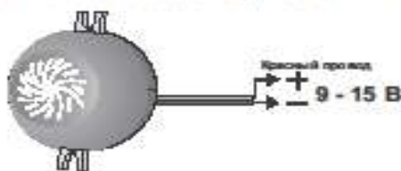
Рис.2 Схема подключения ПКИ-1.
