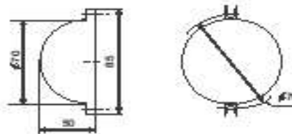
Рис.1. Габаритные и установочные размеры
